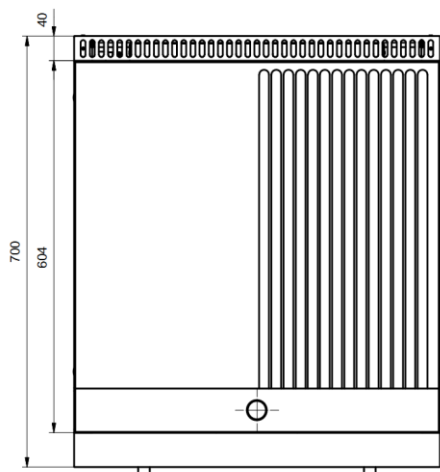
H.1: Kích thước cơ bản thiết bị
